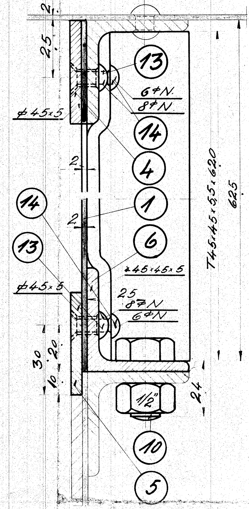
Snit A-A
