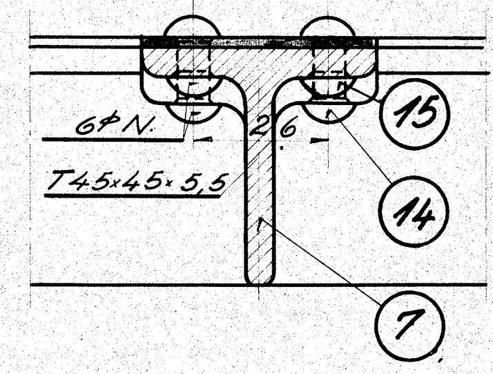
Snit C-C
