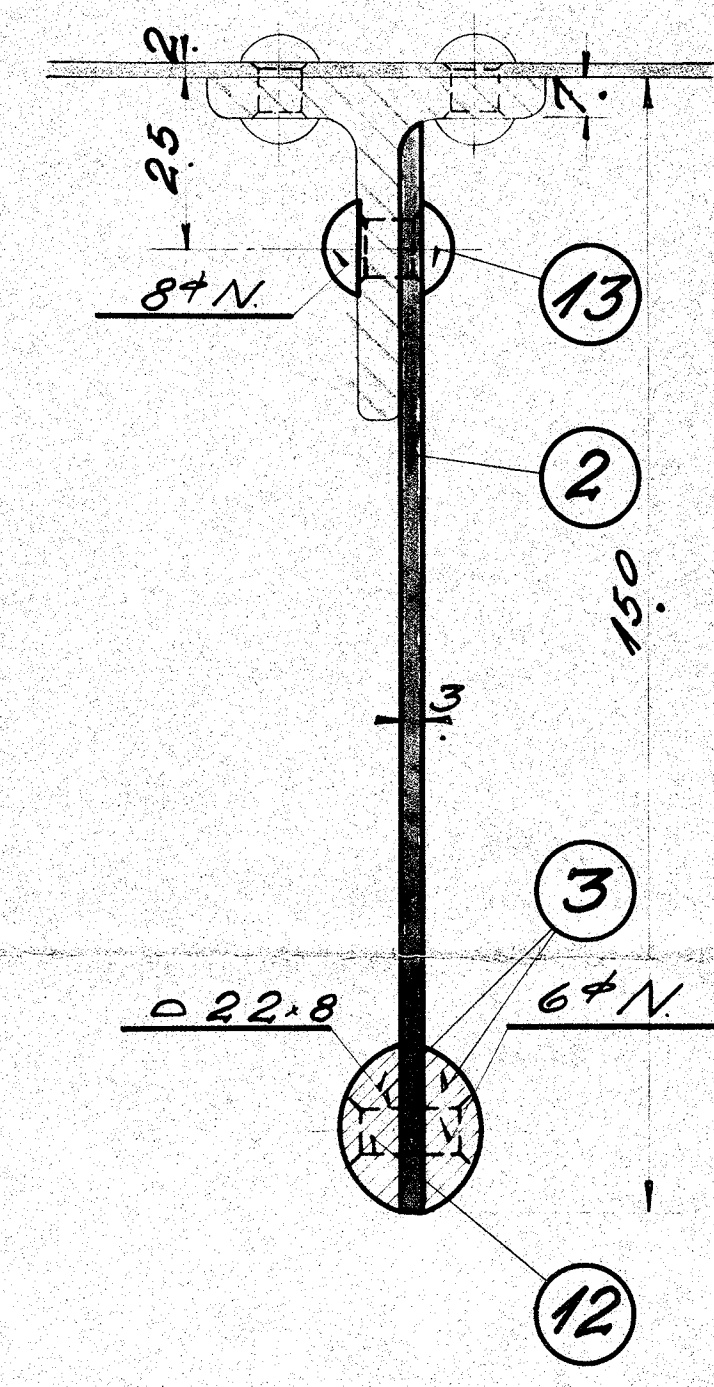
Snit C-C
